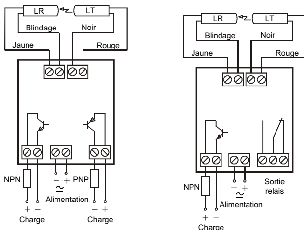
PA 11 D/E 40X Sortie transistor
